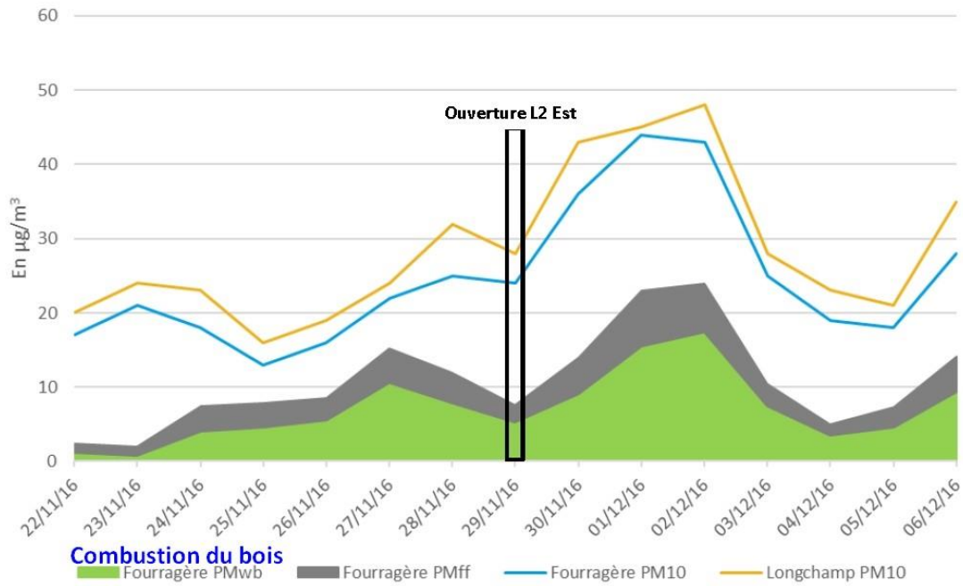
Figure 34 : Evolution des concentrations moyennes journalières en PM 10 , PM wb et PM ff à Marseille / Fourragère 7 jours avant et après l'ouverture de la L2 Est
