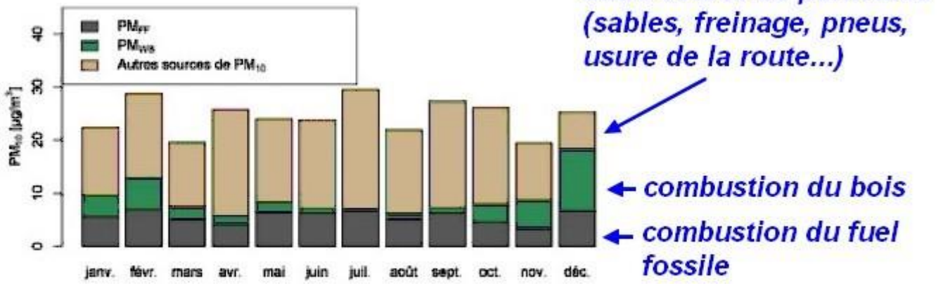
Figure 16: Moyennes mensuelles des concentrations en PM 10 et des fractions issues de la combustion de bois et de la combustion de fuel fossile
